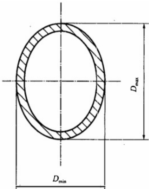
图 4 圆度
