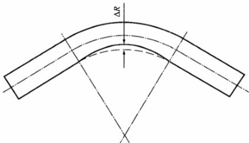
图 11 弯曲半径检测方法
