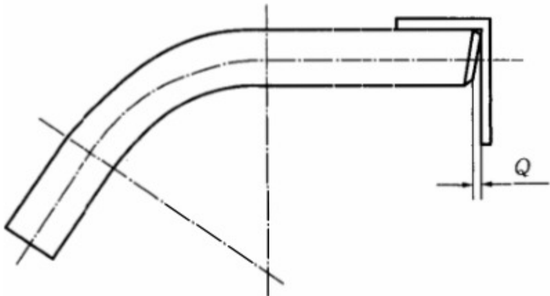
图 13 端面垂直度检测方法
