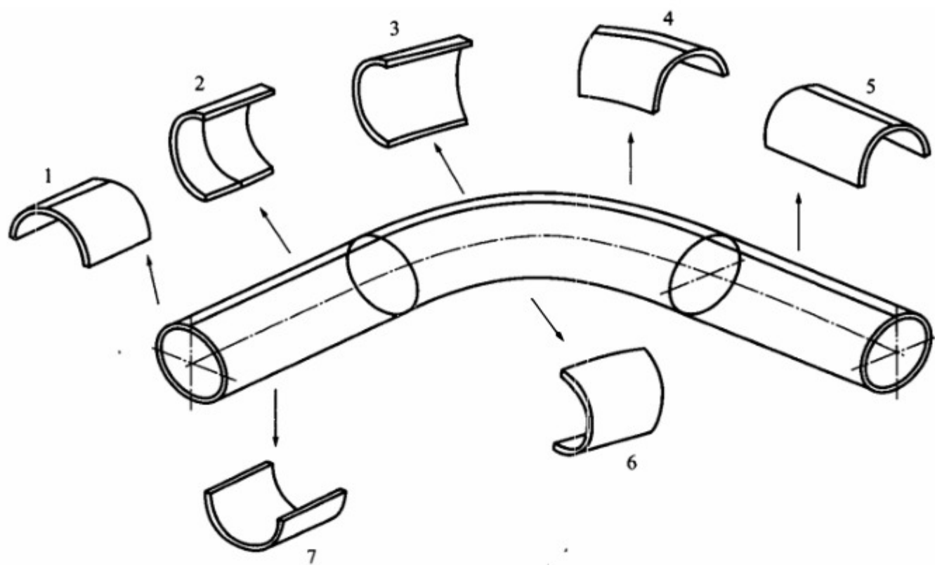
1—直段焊缝；2—过渡区外弧侧；3—外弧侧；4—弯曲区焊缝；5—过渡区焊缝；6—内弧侧；7—直段
