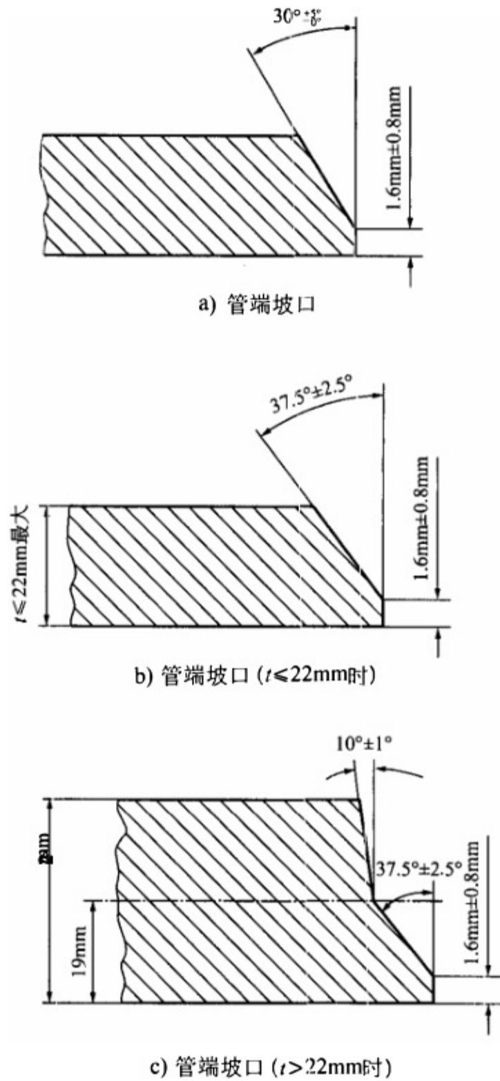
图 9 管端坡口
