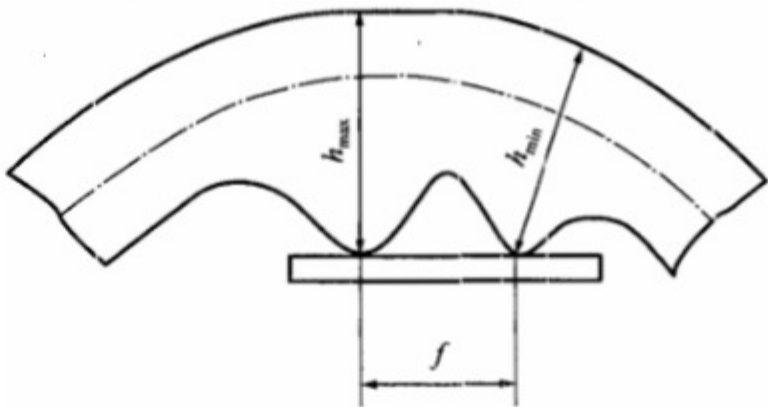
图 12 波浪度和波浪间距检测方法
