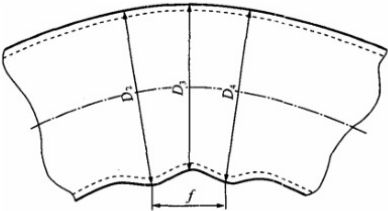
图 3 波浪度与波浪间距测量
