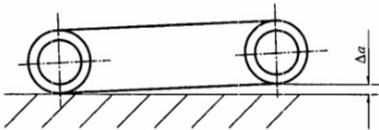
图 6 弯管平面度
