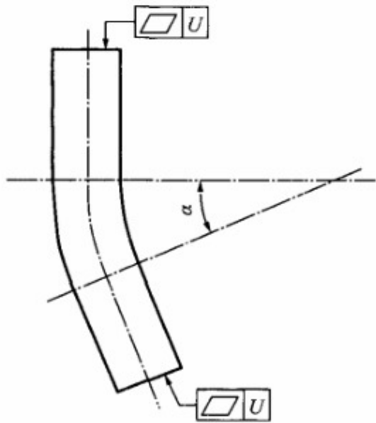
图 8 端面平面度
