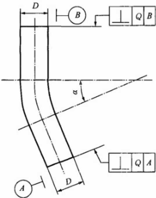
图 7 弯管端面垂直度
